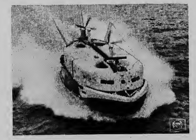
E aparato aki, SR.N3 ta e hovercraft mas grandi y mas potente qu a ser construi. Durante prueba nan rita laman na Inglaierra, eia alcanza un velocidad di 90 milla pa ora.
